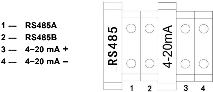
Analyzer wiring
